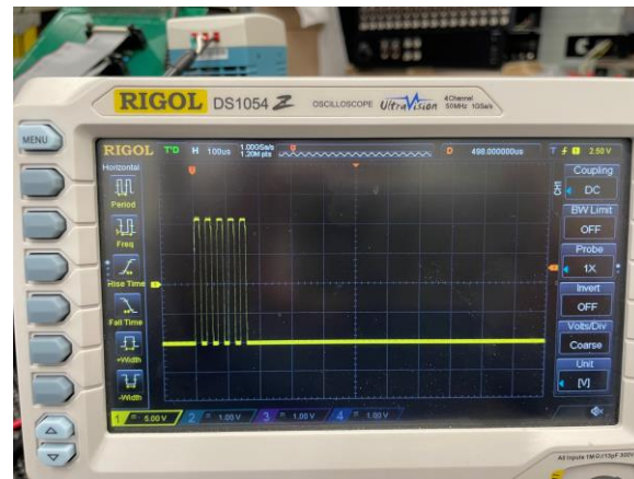
600 baud
