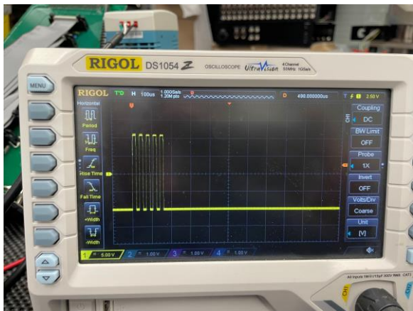
2400 baud
