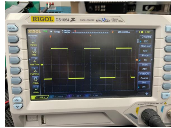
4800 baud
